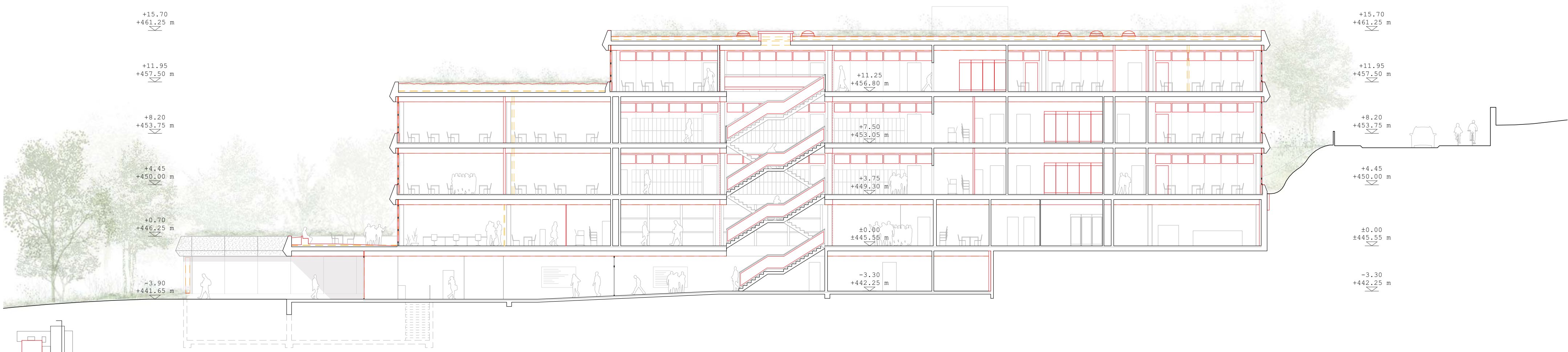
Coupe CC 1:200
