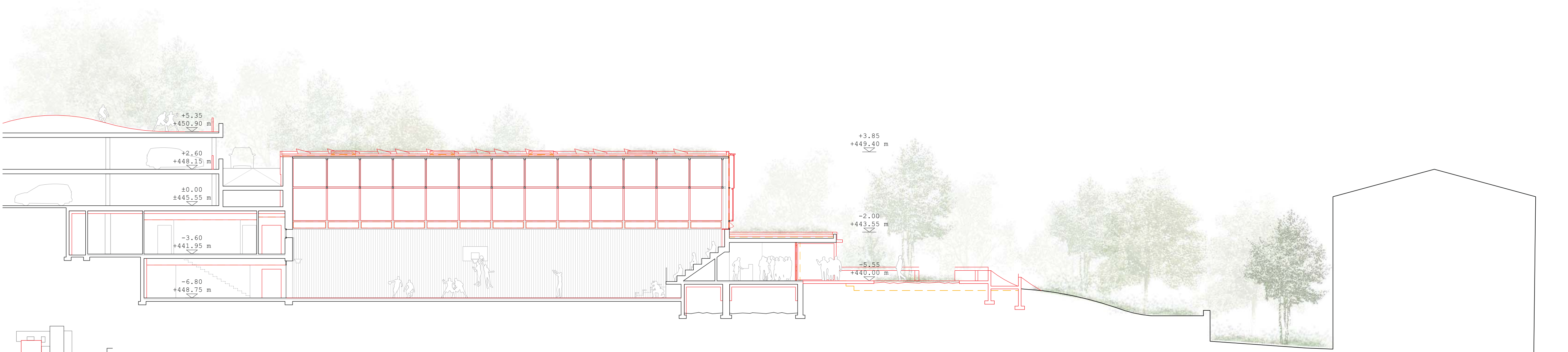
Coupe DD 1:200
