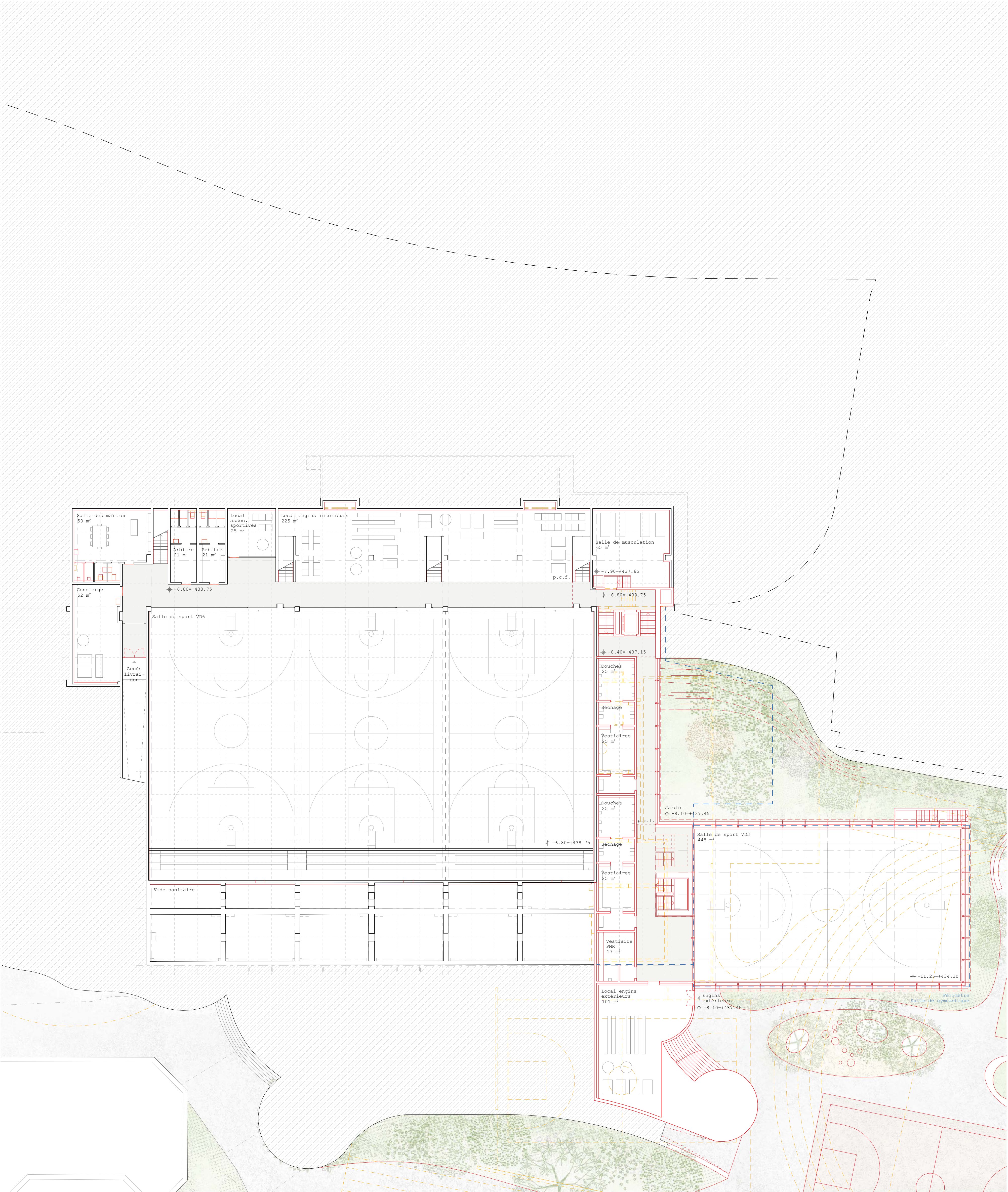
Sous-sol -1 salle de gym 1:200
