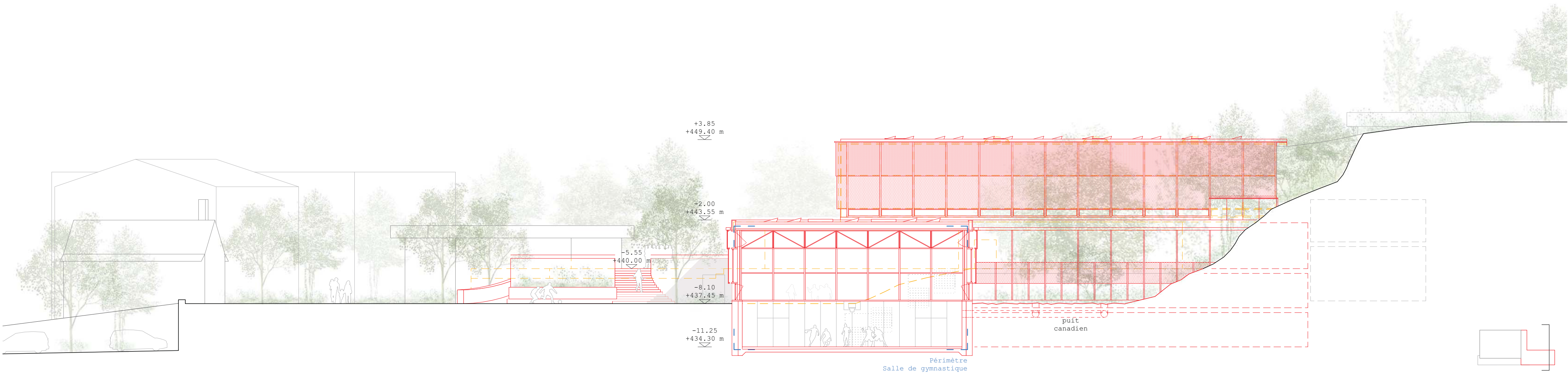
Coupe FF 1:200
